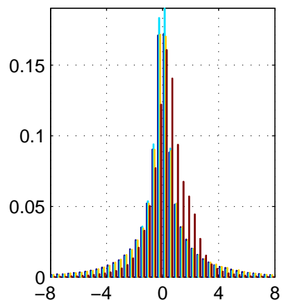
High lat., sunlit
