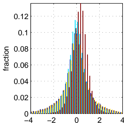
Low lat., sunlit
