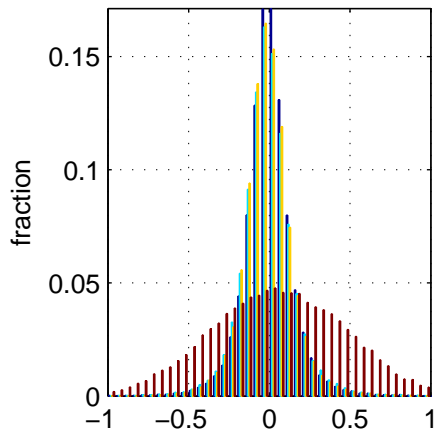
Low lat., dark
