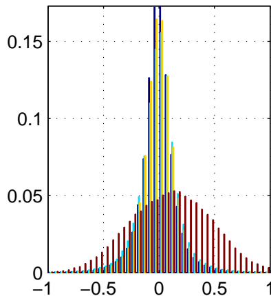
Mid lat., dark
