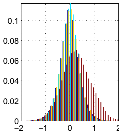
Mid lat., sunlit
