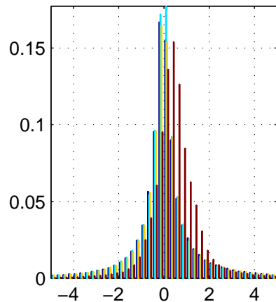
High lat., dark
